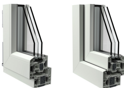
Telaio ad Elle (vista interna ed esterna)
